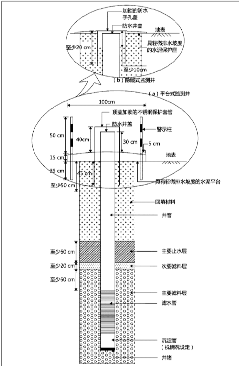
图 D.0.1 地下水监测井井身结构图
